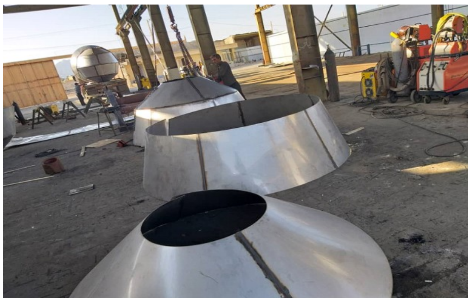
ساخت مخازن کراژنیک - جداره داخلی از جنس SS-304L
